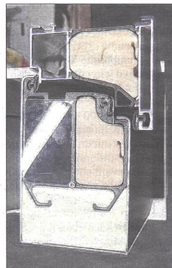
Coupe d'un montant de porte blindée. Photo ER/Philippe PIOT
